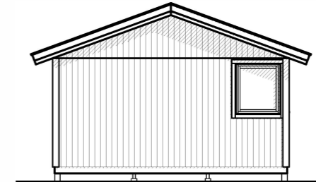
FASAD MOT
